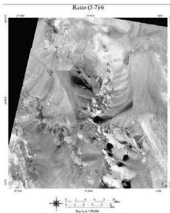
شکل ۴. نسبت باندهی مرکب (B5+B7)/B6 جهت بارزسازی زون فیلیک
