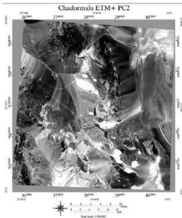
شکل ۱۱. تصویر PC2 از آنالیز مؤلفه‌های اصلی استاندارد سنجنده ETM+ (کانی‌های هیدروکسیل مناطق روشن)
