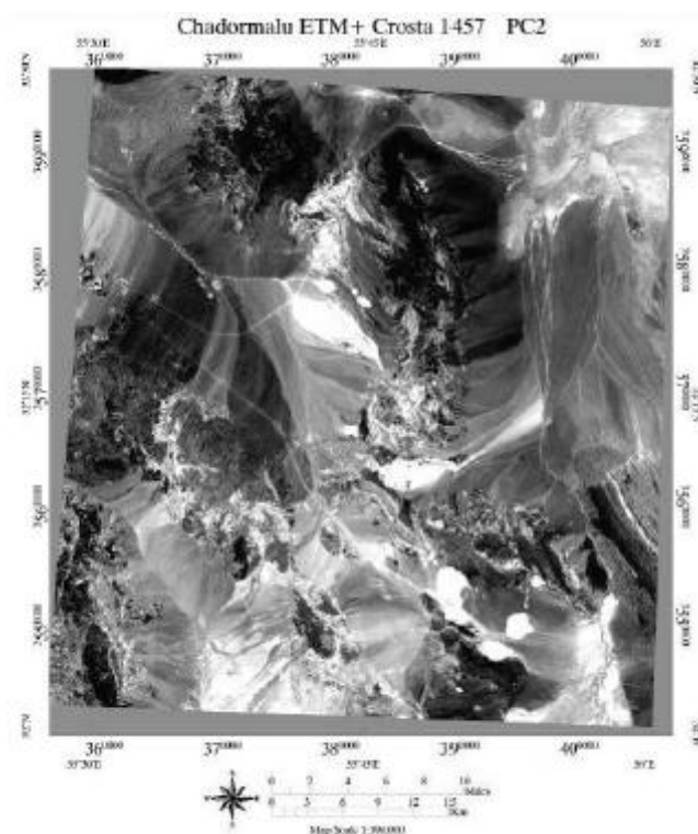
شکل ۱۲. تصویر PC2 از آنالیز PCA باندهای ۱، ۴، ۵ و ۷ سنجنده ETM + (کانی‌های حاوی هیدروکسیل مناطق روشن)
