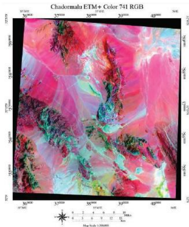
شکل ۶. تصویر رنگی کاذب سنجنده ETM + در منطقه مورد مطالعه (RGB=۷۴۱)
