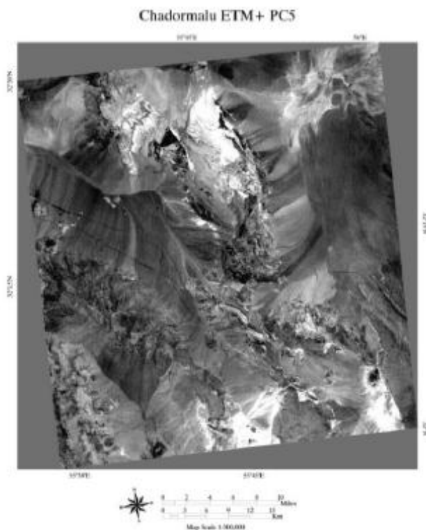
شکل ۱۰. تصویر PC5 از آنالیز مؤلفه‌های اصلی استاندارد سنجنده ETM+ (اکسیدهای آهن مناطق روشن)
