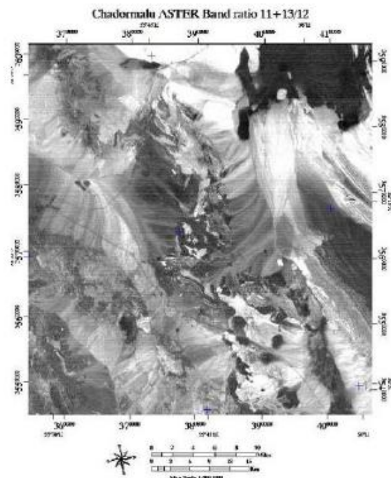
شکل ۵ نسبت باندهی مرکب (B11+B13)/B12 جهت بارزسازی ماسه سنگ
