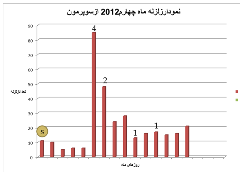
شکل ۴- نمودار زمین‌لرزه‌های با بزرگای بیش‌تر از ۵/۰ ماه آپریل ۲۰۱۲ شروع از روز وقوع ابرماه و زمین‌لرزه‌های با بزرگای بیش از ۷/۰ در بالای نمودارها، روز نوشته شده است. ابرماه بانماد S نشان داده شده است.
