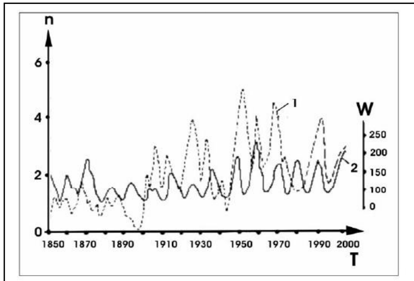
شکل ۱- نمودار مقایسه رابطه‌ی میان فعالیت خورشیدی و فعالیت آتشفشانی، در نمودار منحنی ۱ (نقطه چین) فعالیت آتشفشانی و منحنی ۲ (خط پر) فعالیت خورشیدی را نشان می‌دهد (خاین و خلیف، ۲۰۰۸).
