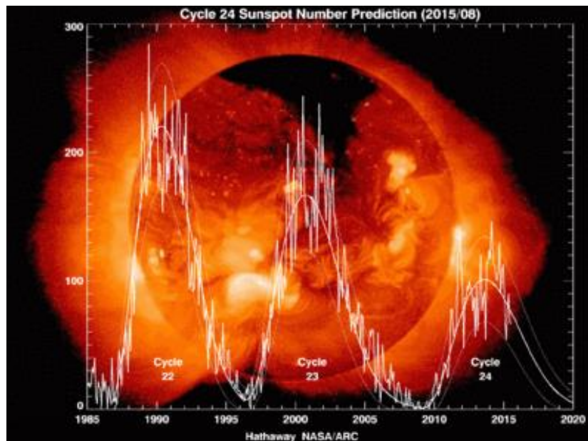
شکل ۵ - نمودار دوره‌های فعالیت خورشیدی از سال ۱۹۸۵ تا ۲۰۱۵ که شامل سه دوره ۱۱ ساله فعالیت خورشیدی است.
