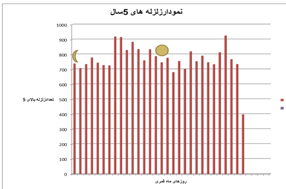
شکل ۳- نمودار مجموع زمین‌لرزه‌های با بزرگای بیش‌تر از ۵/۰ سال‌های ۲۰۱۱ تا ۲۰۱۵ برحسب شروع از ماه نو، در اینجا ماه نو و ماه کامل بانماد دایره و هلال ماه مشخص شده است. هم‌بستگی بیش‌تری پس از ماه نو در مقایسه با ماه کامل دیده می‌شود.
